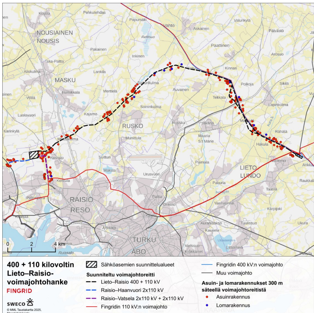
Kuva 5-15. Asuin- ja lomarakennukset 300 metrin säteellä suunnitelluista voimajohtoista.
